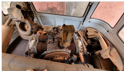
MOTOR COMPARTIMENTO
