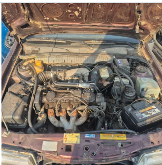
MOTOR COMPARTIMENTO
