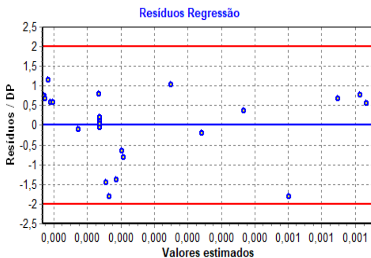
Resíduos da Regressão Linear
