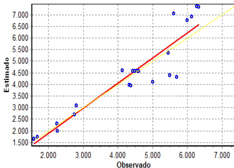
Aderência Observado x Estimado - Regressão Linear na forma direta
